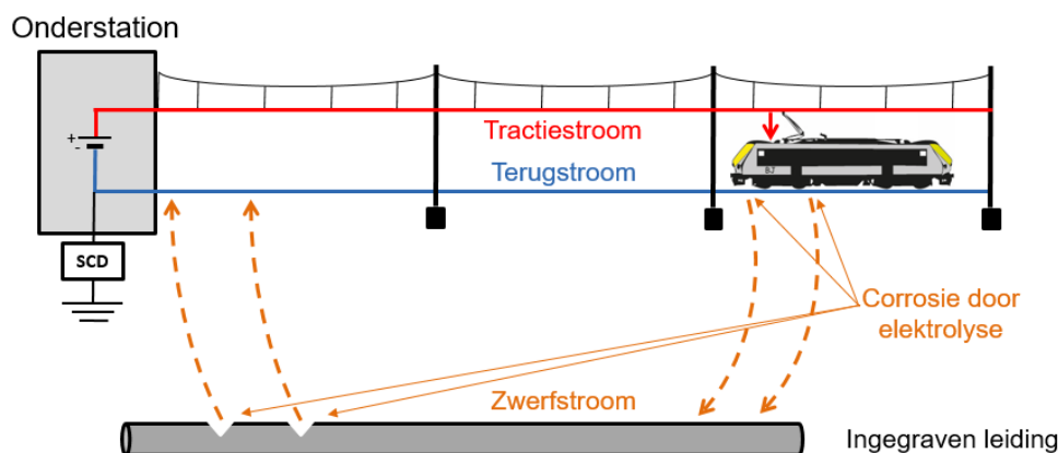
Afbeelding 2.27 - Zwerfstroom en elektrolytische corrosie
