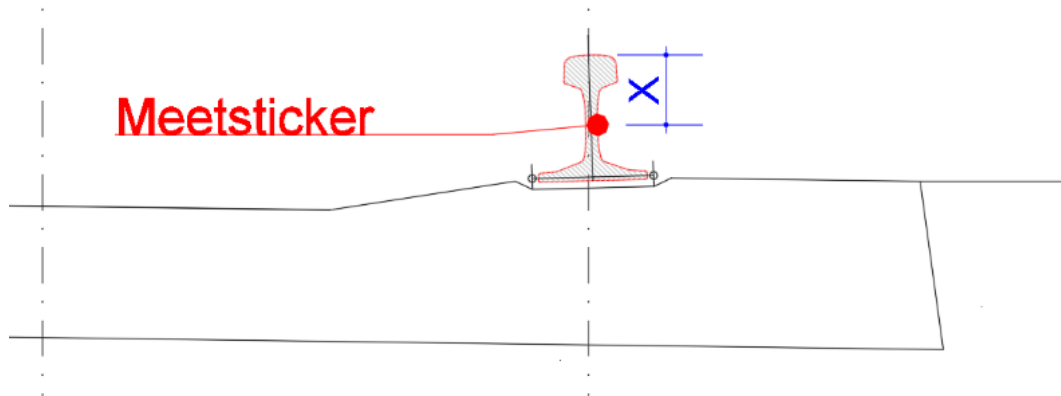
Afbeelding 2.11 - Plaatsing van de meetsticker
