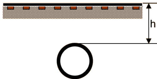
Afbeelding 2.7 - Minimale dekking
