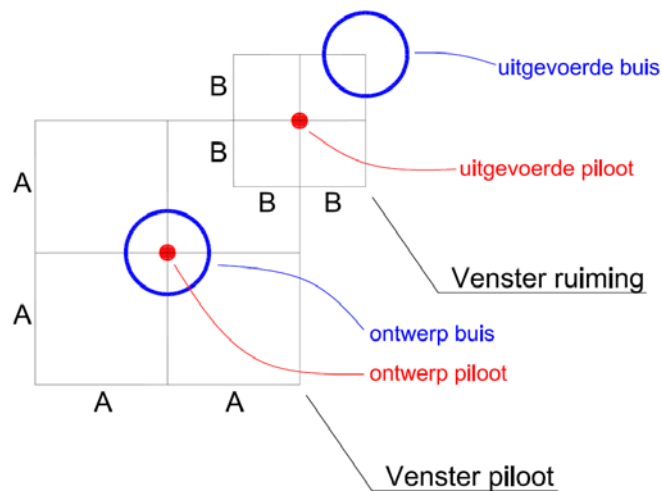
Afbeelding 2.23 – Toleranties venster piloot-ruiming
