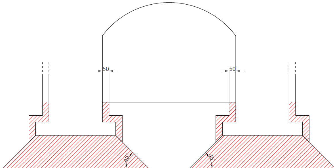
Afbeelding 2.4 - zone not aedificandi onder de invloedszone van de funderingen van een kunstwerk
