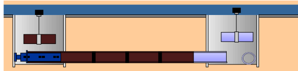
Afbeelding 2.20 - Pilotstangendoorpersing muren productbuis
