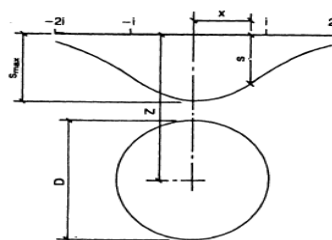
Afbeelding 2.21 - karakteristieken van de waarschijnlijkheidskromme als zettingstrog boven cirkelvormige tunnel
