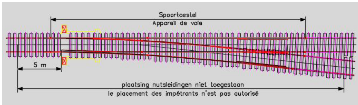
Afbeelding 2.2 - Verboden werkzone - spoortoestel
