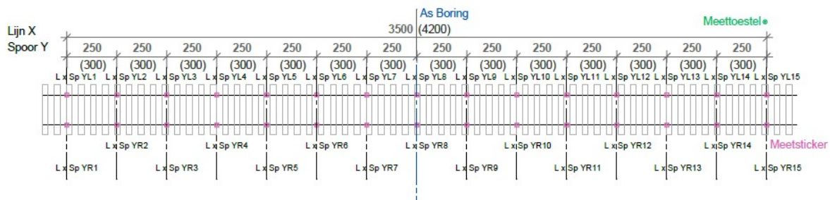
Afbeelding 2.10 - Werkzone bovenaanzicht
