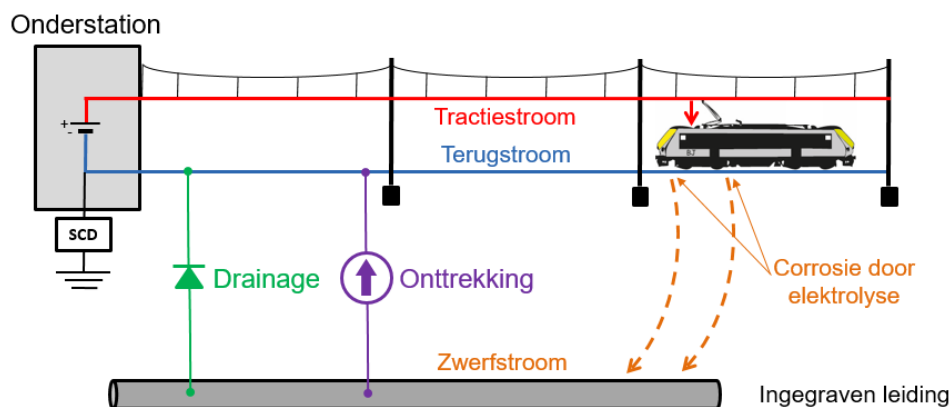
Afbeelding 2.28 - Zwerfstroom en kathodische bescherming
