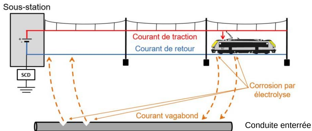
Figure 2.27 : Courants vagabonds et corrosion électrolytique
