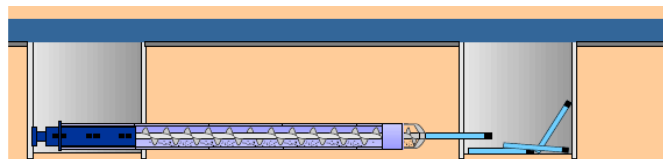
Figure 2.19 : Fonçage avec tige pilote –curage à la tarière
