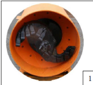
Figure 2.15 : Bouclier ouvert(1)
