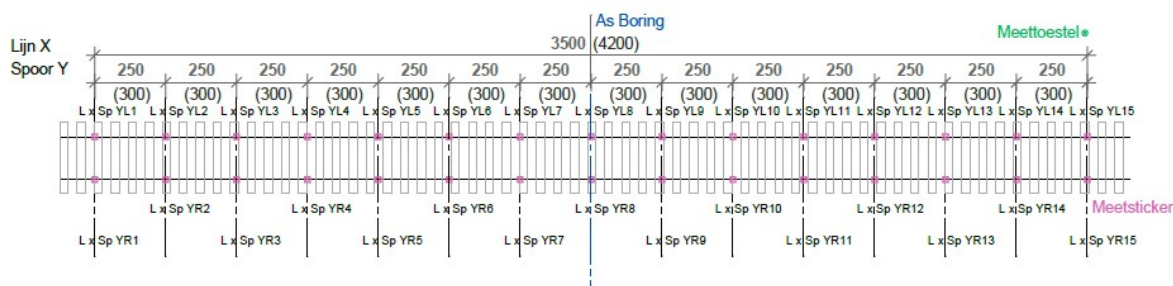
Figure 2.10 - Zone de travail - vue en plan
