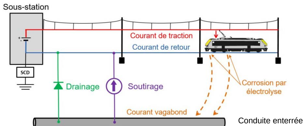
Figure 2.28 : Courants vagabonds et protection cathodique
