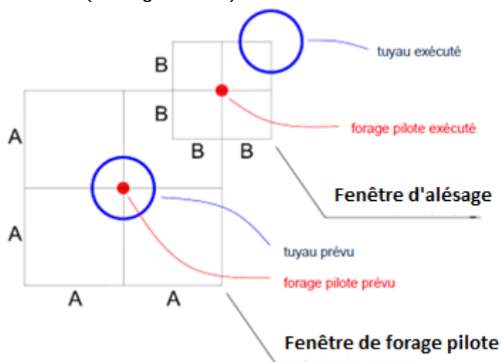
Figure 2.23 : Tolérances fenêtre pilote-alésage
